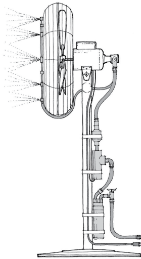
Fig. 09: Misting fan
