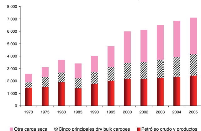
Gráfico 3 COMERCIO MARÍTIMO INTERNACIONAL, 1970-2005
