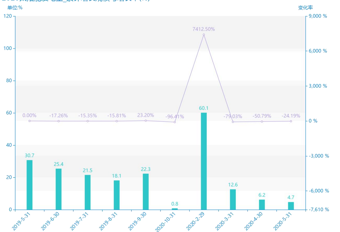
2019-2020太阳能发电量_累计增长规模与增长率(%)
