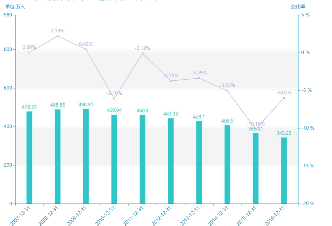
2007-2016城市液化石油气用气人口规模与增长率(万人)
