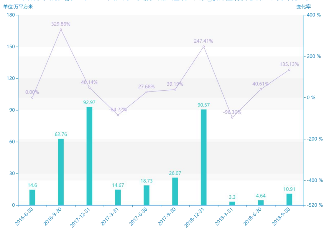
2016-2018国有及国有控股建筑业企业其他商业及服务用房竣工面积_累计规模与增长率(万平方米) —○— 增长率
