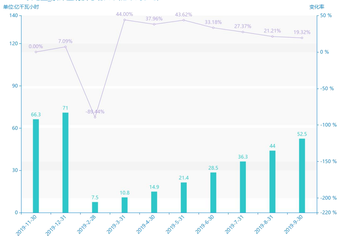
2019-2019发电量_累计值规模与增长率(亿千瓦时)
