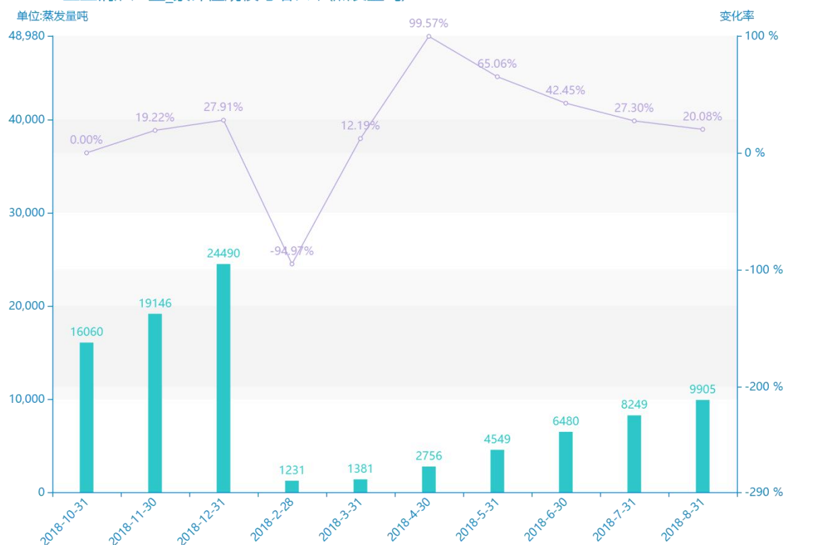
2018-2018工业锅炉产量_累计值规模与增长率(蒸发量吨)
