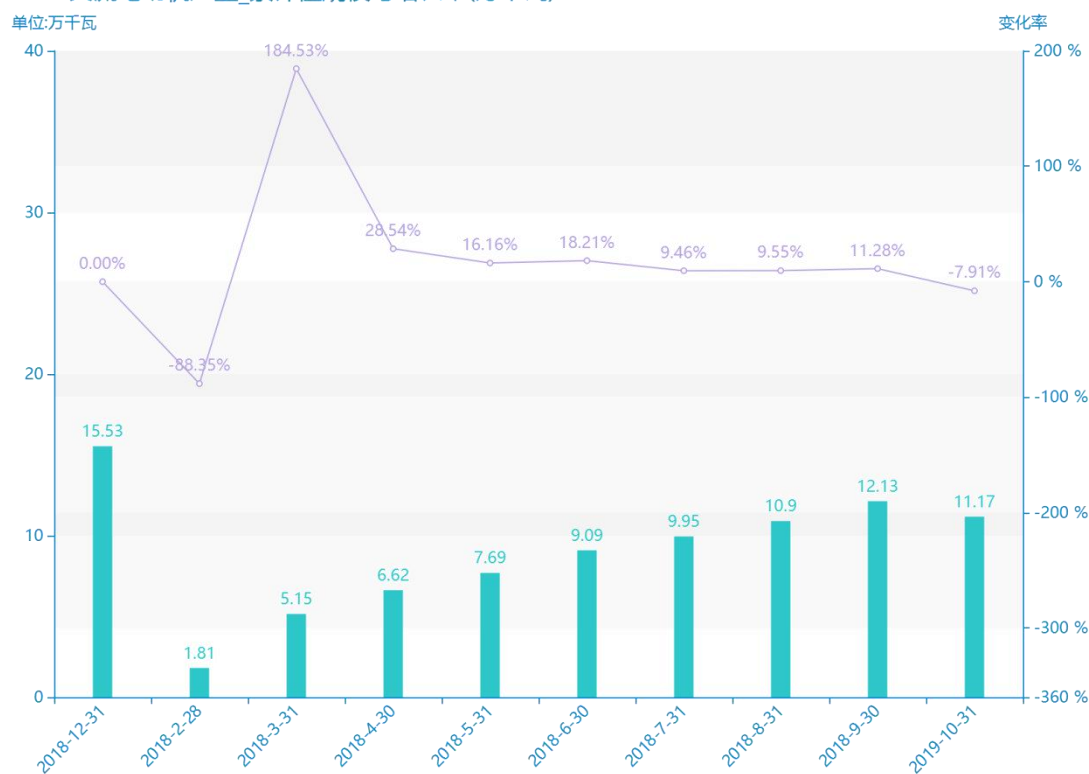
2018-2019交流电动机产量_累计值规模与增长率(万千瓦)
