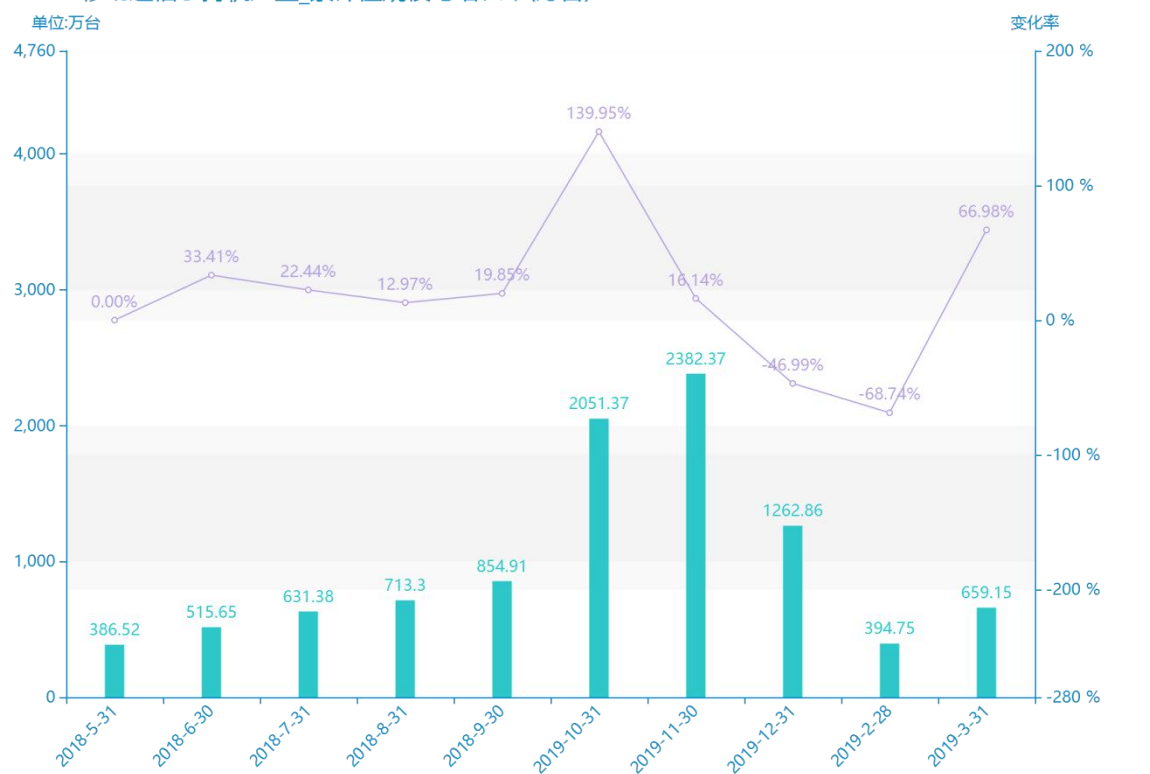
2018-2019移动通信手持机产量_累计值规模与增长率(万台)
