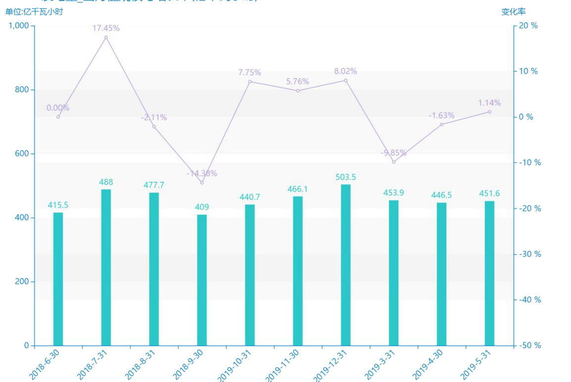
2018-2019发电量_当月值规模与增长率(亿千瓦小时)
