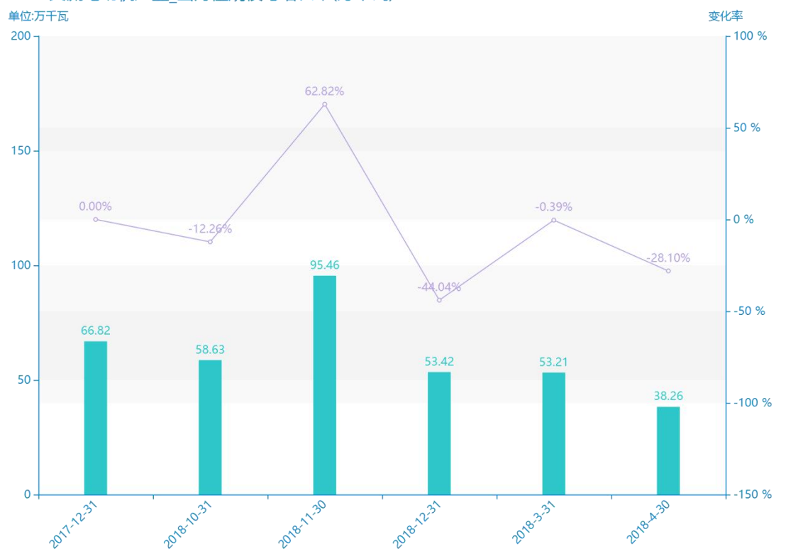
2017-2018交流电动机产量_当月值规模与增长率(万千瓦)
