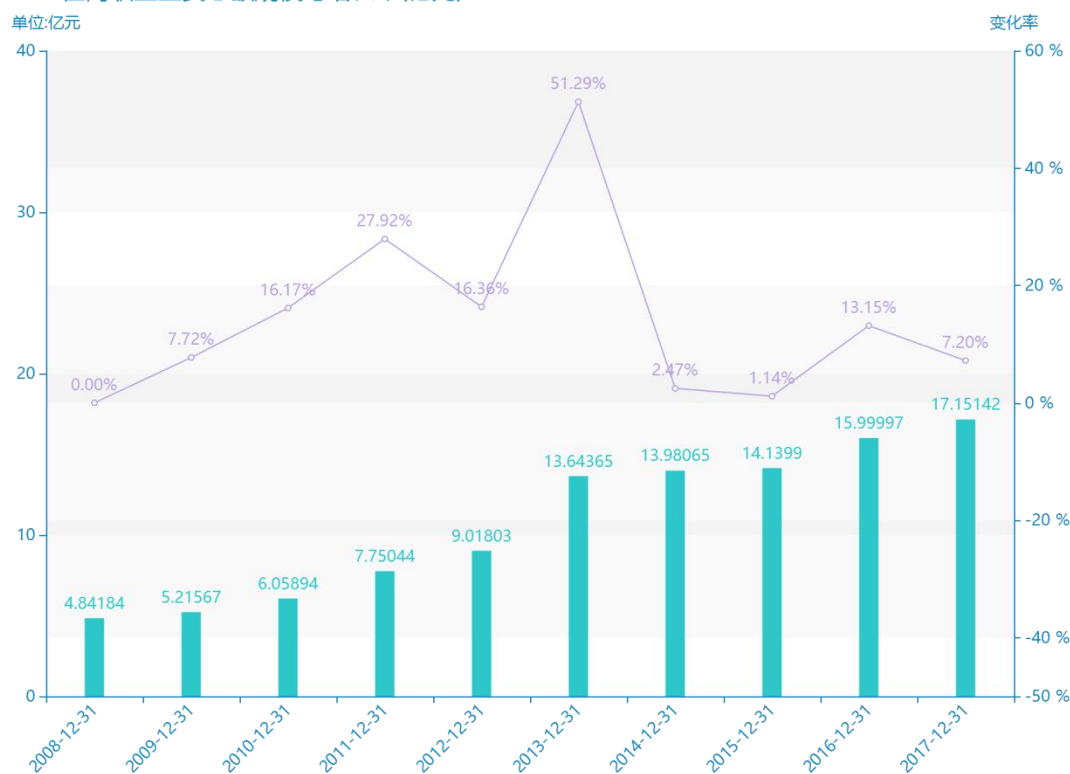
2008-2017在岗职工工资总额规模与增长率(亿元)
