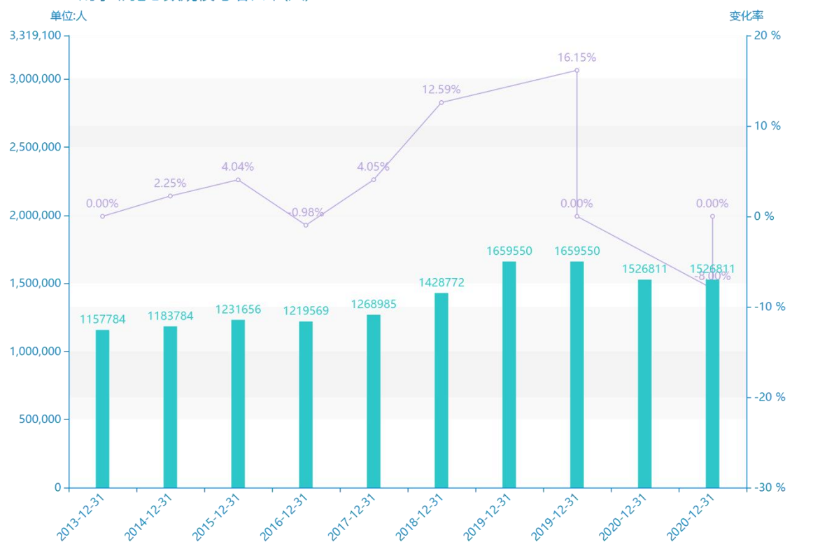
2013-2020刑事罪犯总数规模与增长率(人)
