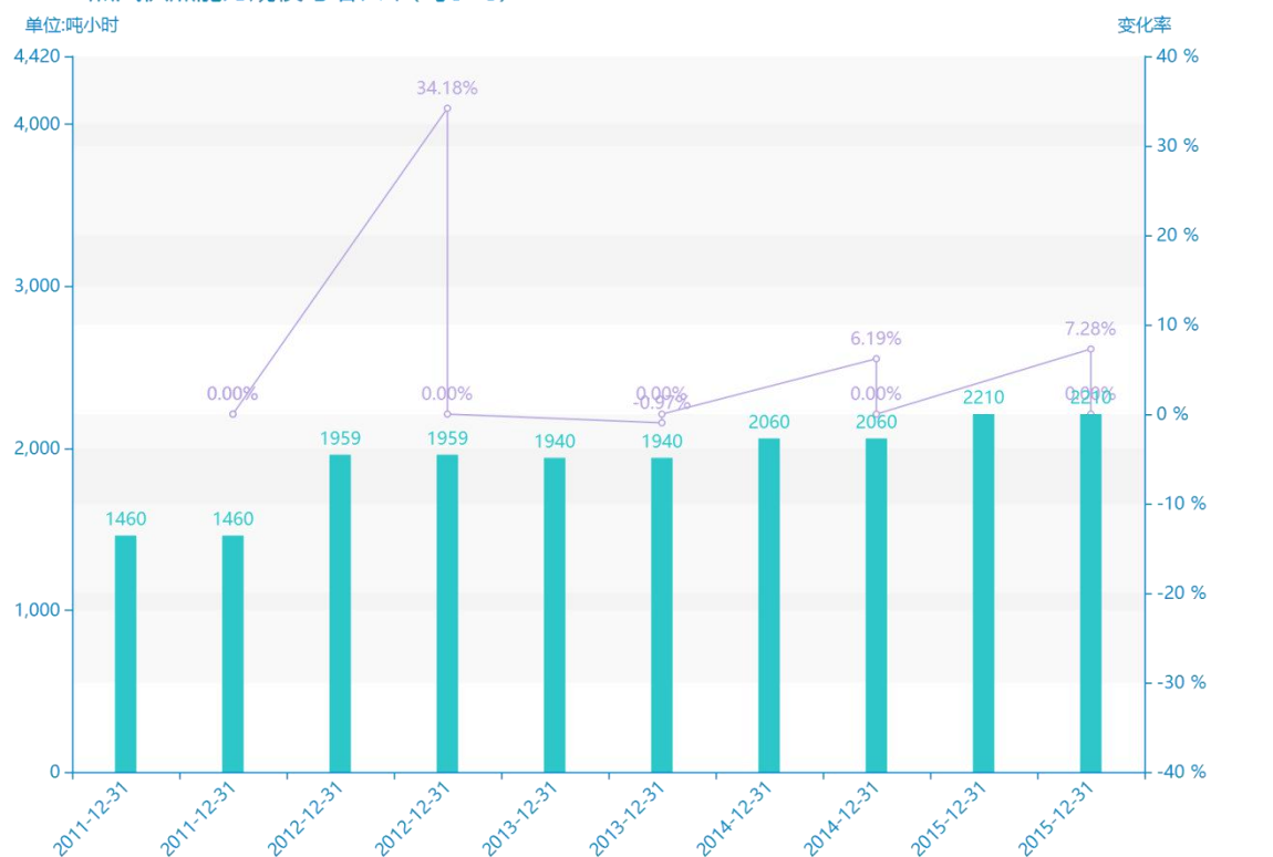
2011-2015蒸汽供热能力规模与增长率(吨小时)
