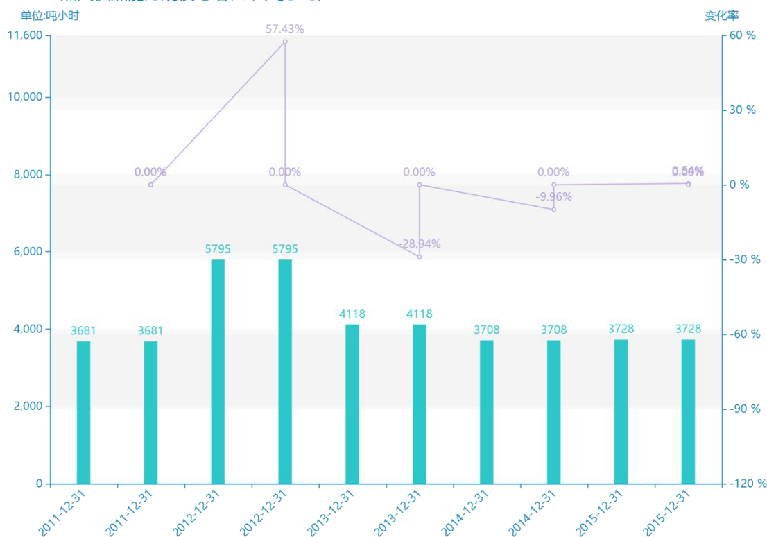
2011-2015蒸汽供热能力规模与增长率(吨小时)
