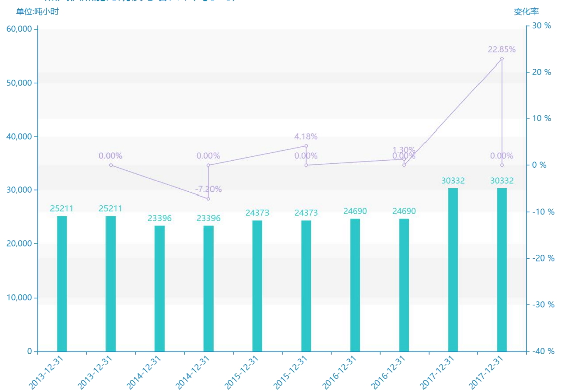
2013-2017蒸汽供热能力规模与增长率(吨小时)
