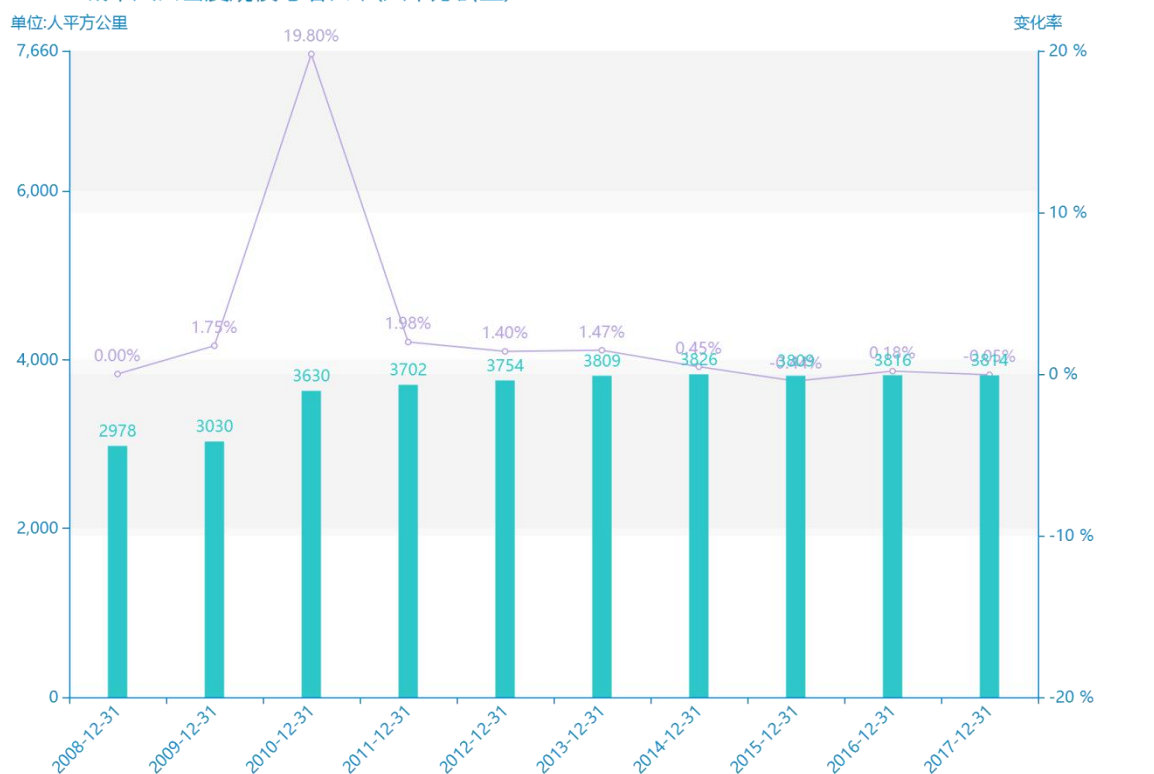
2008-2017城市人口密度规模与增长率(人平方公里)
