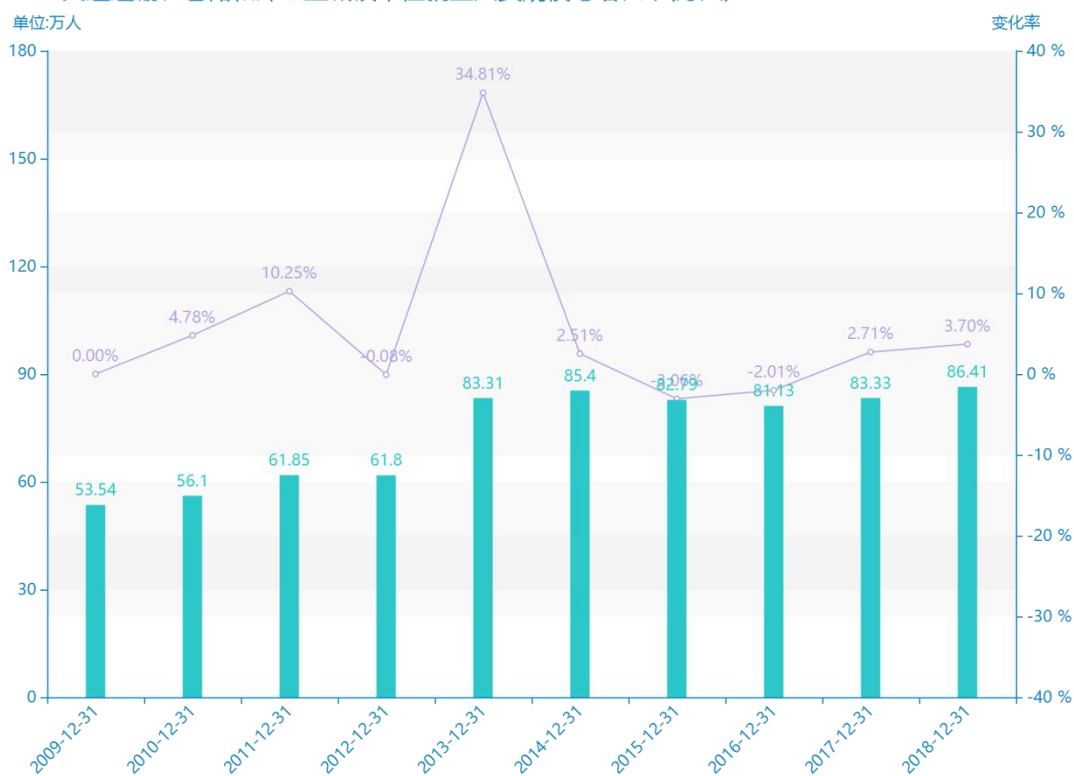
2009-2018交通运输、仓储和邮政业城镇单位就业人员规模与增长率
