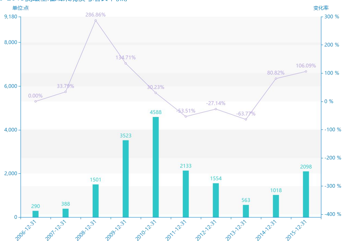
2006-2015测绘基准成果规模与增长率(点)
