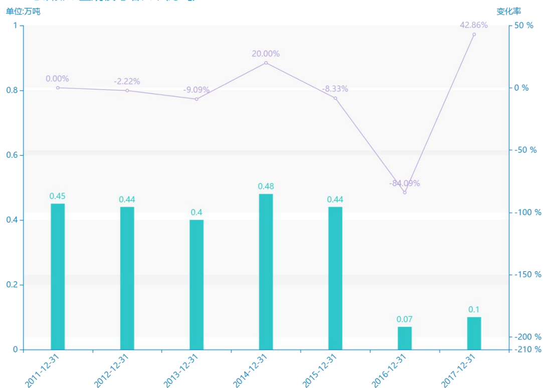
2011-2017总磷排放量规模与增长率(万吨)
