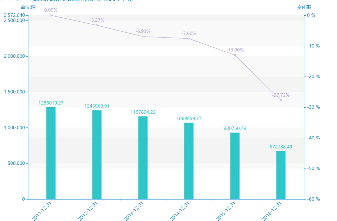
2011-2016氮氧化物排放量规模与增长率(吨)
