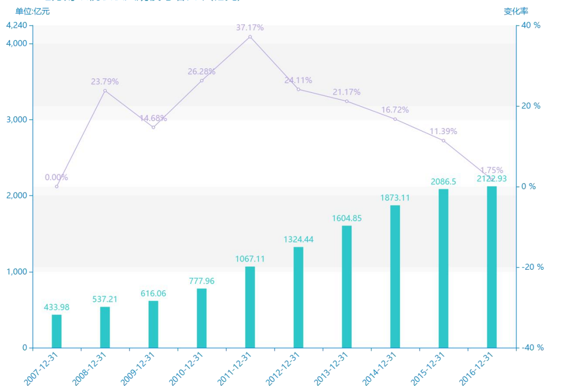
2007-2016地方财政税收收入规模与增长率(亿元)
