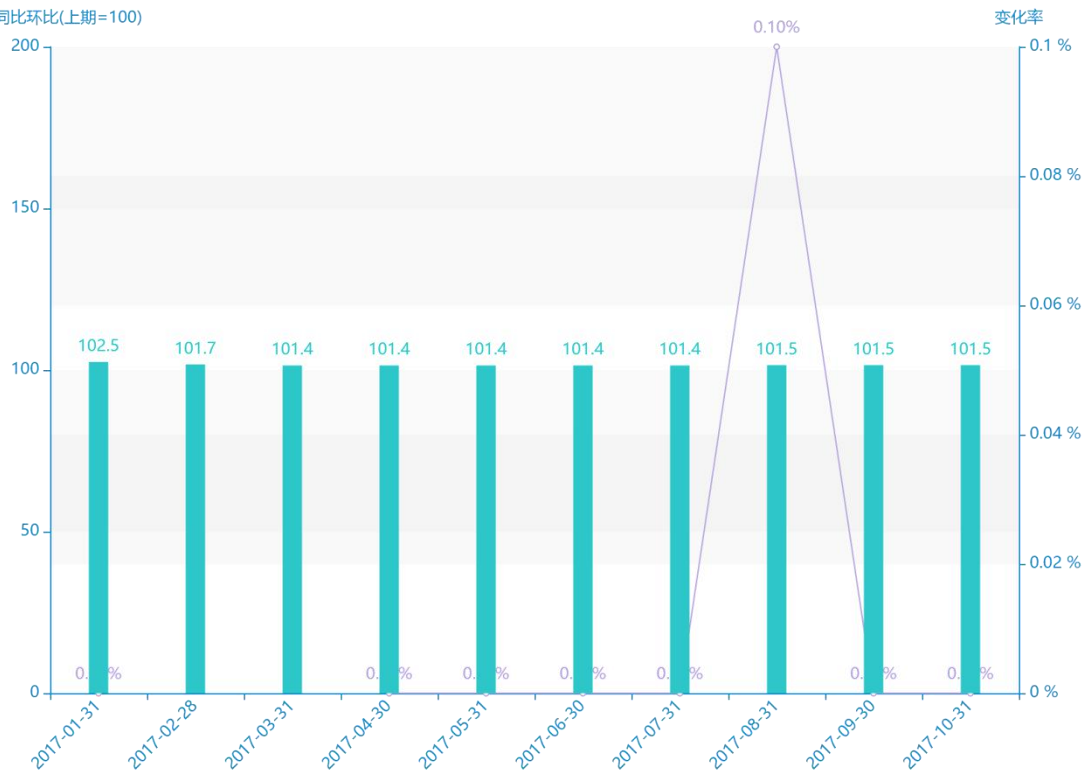
2017-2017居民消费价格指数规模与增长率(同比环比(上期=100))
