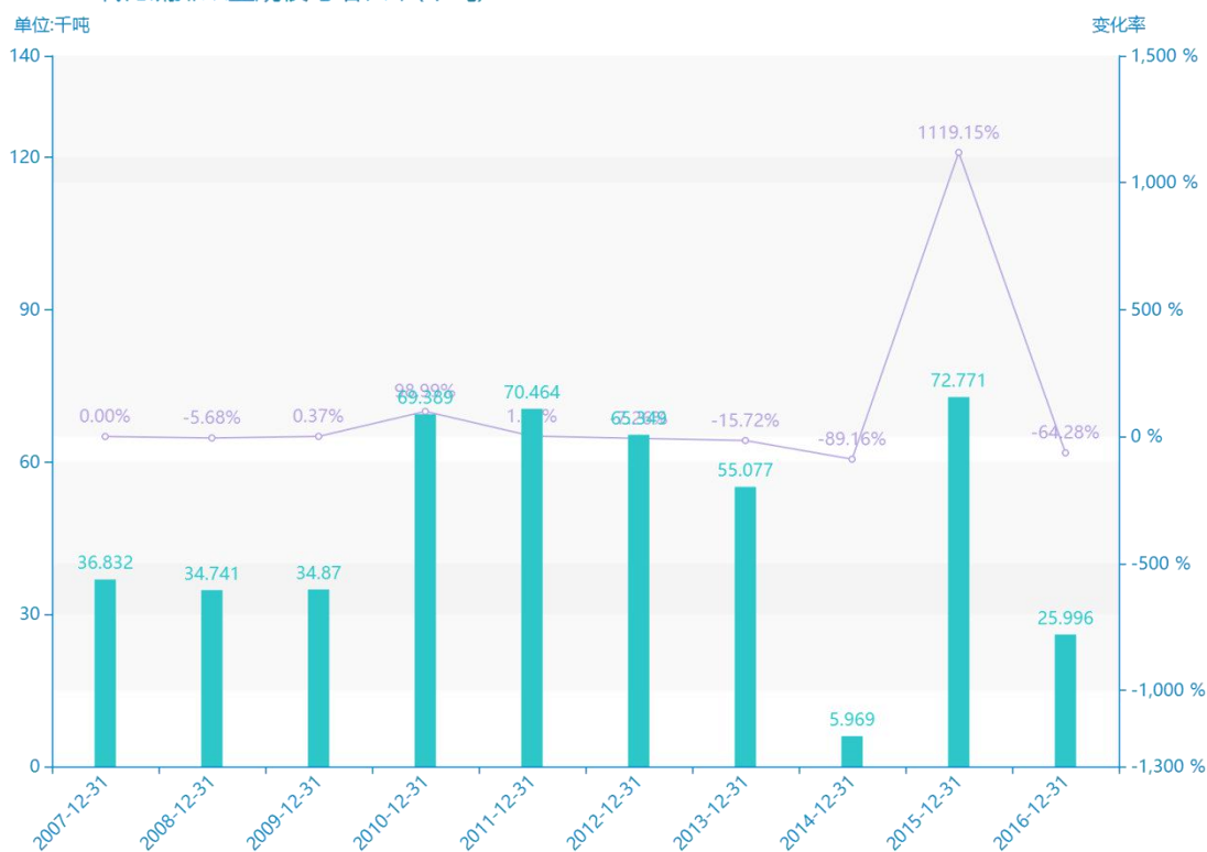
2007-2016二氧化硫排放量规模与增长率(千吨)
