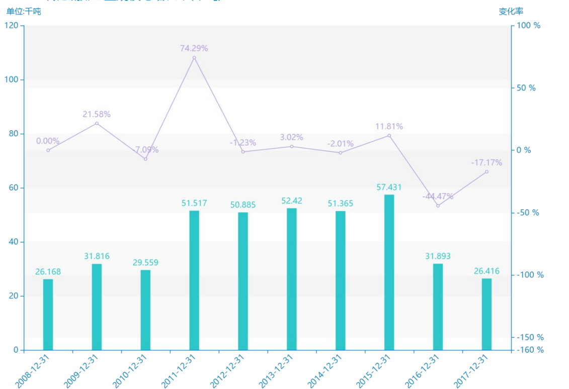
2008-2017二氧化硫排放量规模与增长率(千吨)
