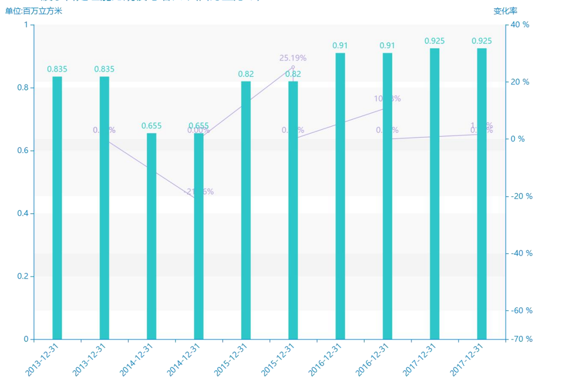
2013-2017废水日处理能力规模与增长率(百万立方米)
