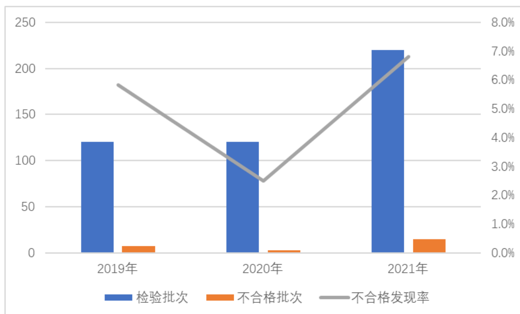
图1 固定式通用灯具产品近3年国家监督抽查情况
