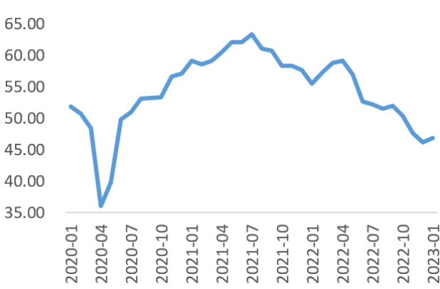
图 4 美国制造业 PMI 走势
