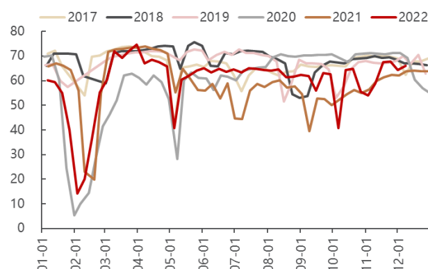
图12：汽车轮胎（半钢胎）开工率上升 (%)
