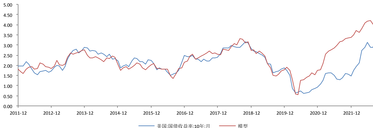
图8：美十债模型
