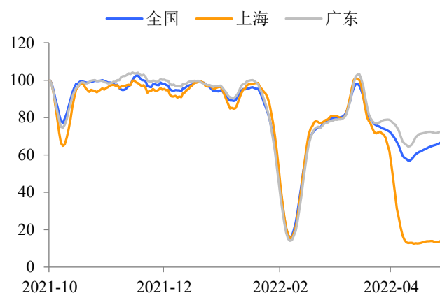
图2: 整车流量指数: 全国, 上海和广东
