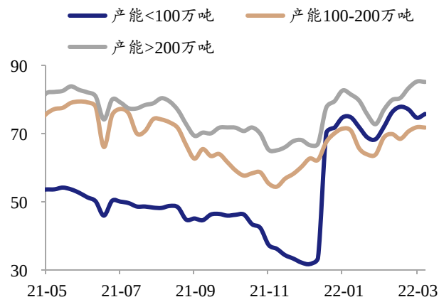
图 6：各产能的焦化企业开工率涨跌互现（%）
