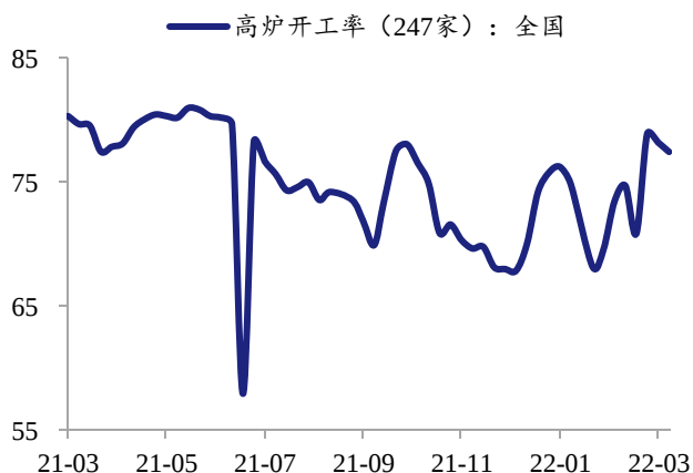
图 5：高炉开工率上行（%）
