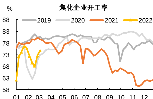
图表8 本周焦化企业开工率 74.8%，环比上升 2.1 个百分点
