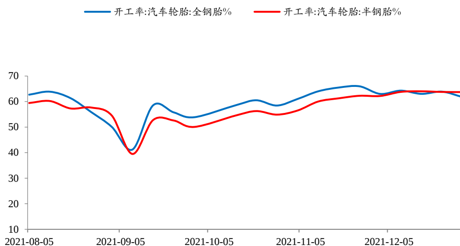
图5： 汽车轮胎开工率略有下降
