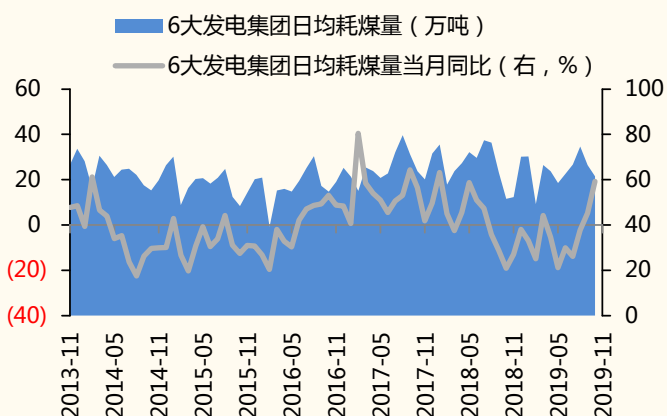
图表 7：10 月以来 6 大发电集团日均煤耗同比涨幅扩大
