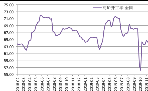
图 9：高炉开工率
