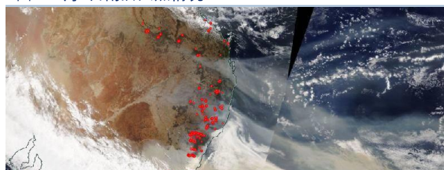
图6: 1月5日雨后火点情况
