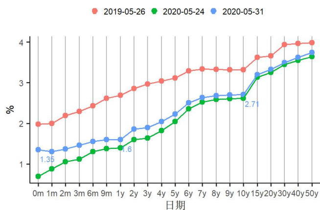
图9 国债到期收益率曲线
