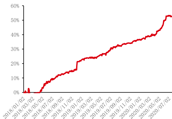
图 8：VN30 套利
