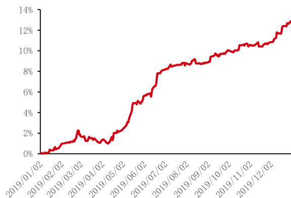
图 7：IC 套利
