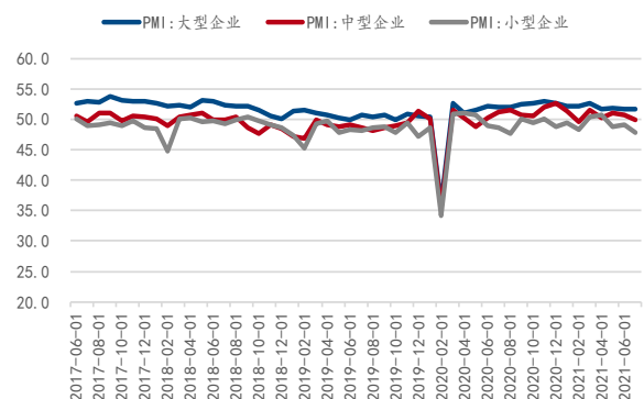
图 6：小企业经营压力凸显
