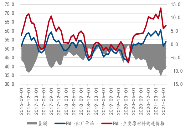
图 4：出厂、原材料购进价格纷纷反弹
