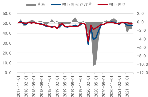
图 3：进出口纷纷回落
