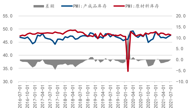
图 5：产成品、原材料库存剪刀差手指标
