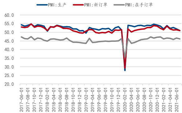
图 2：供需两端纷纷回落
