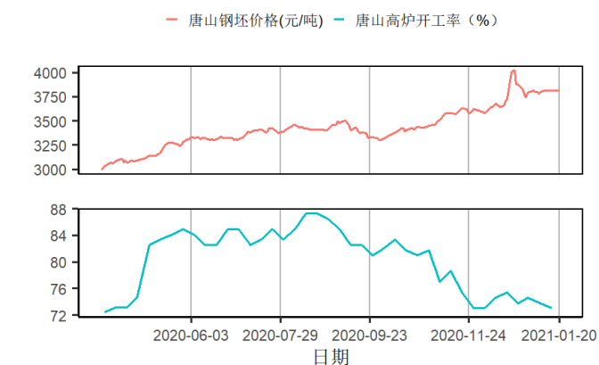
图10 截至2021年01月20日的一周，唐山钢坯价格周环比维持3810元/吨
