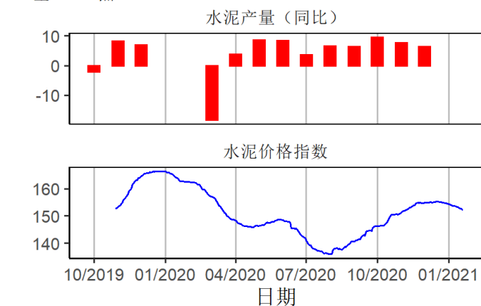
图11 截至2021年01月20日的一周，全国水泥价格指数下跌0.98点至152.25点
