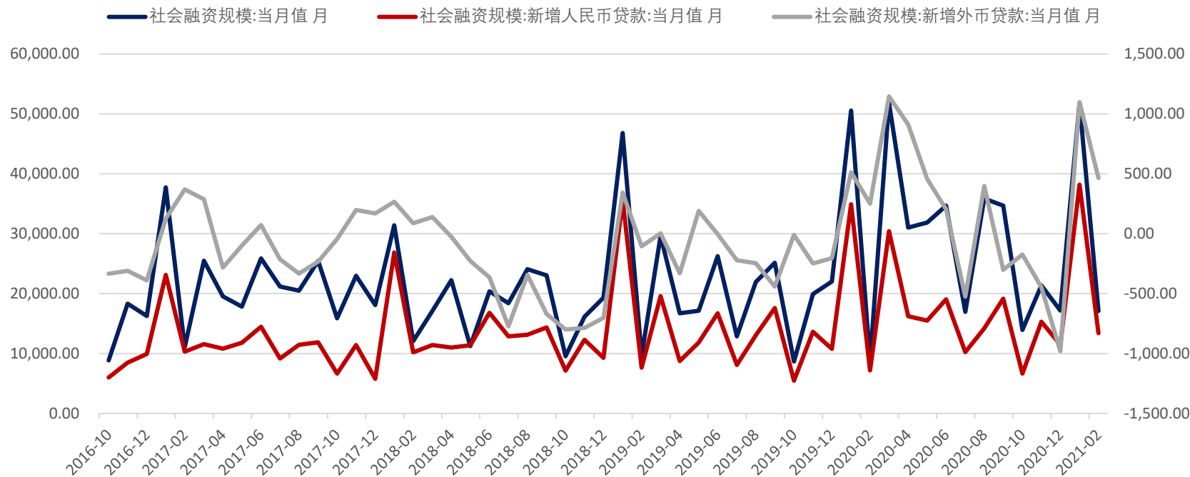
图：社融数据
