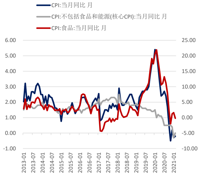
图：CPI数据
