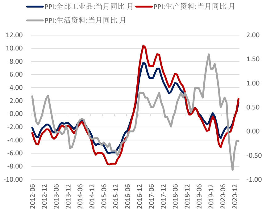
图：PPI数据
