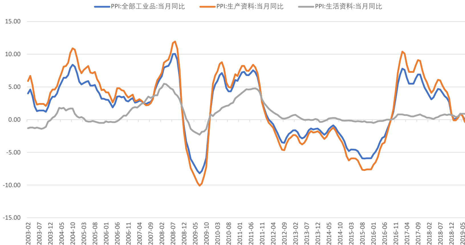
图：PPI
