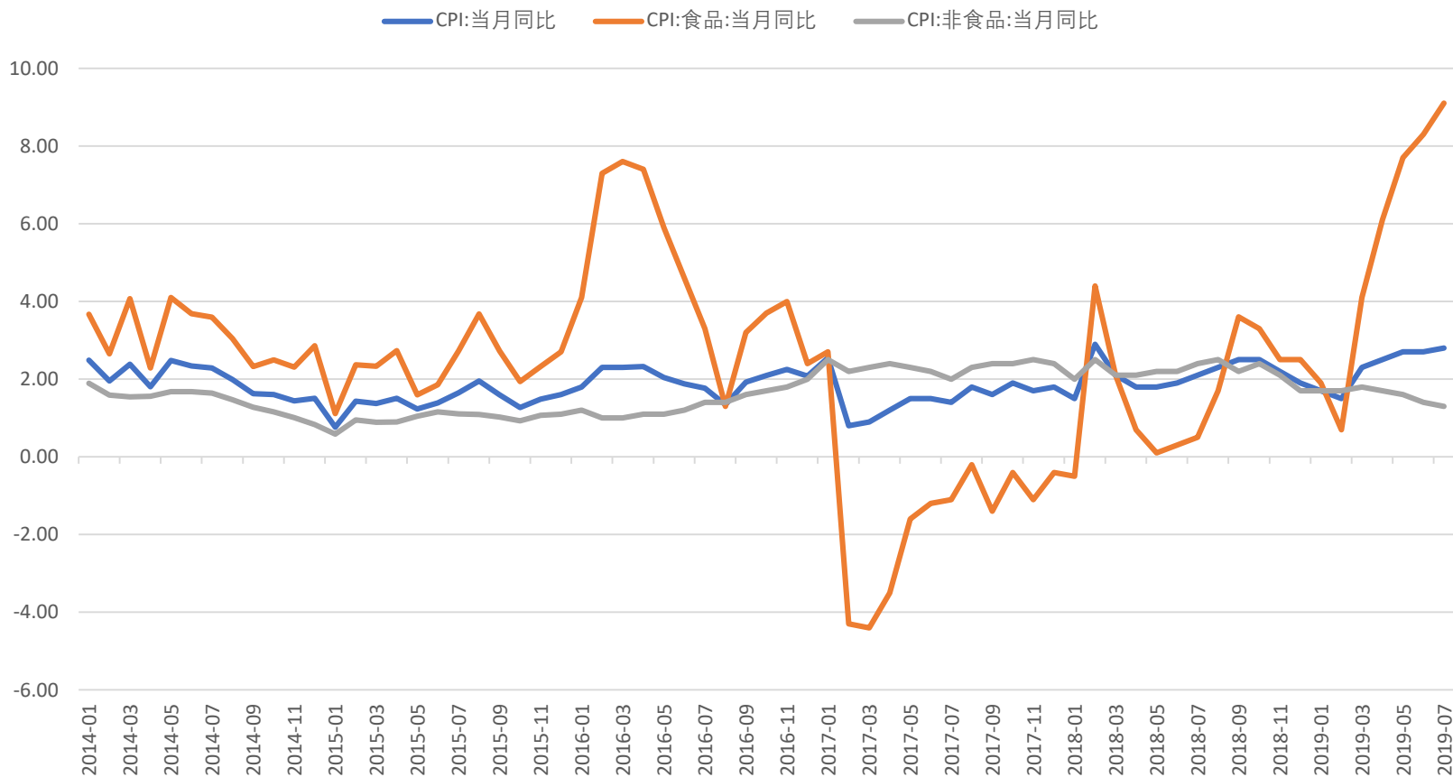
图：CPI
